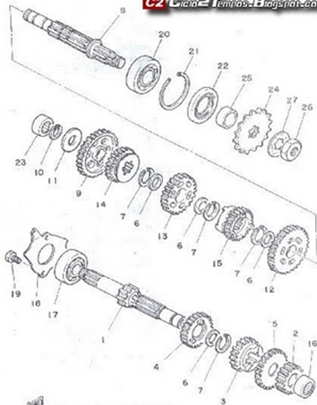
Transmissão Rd135
