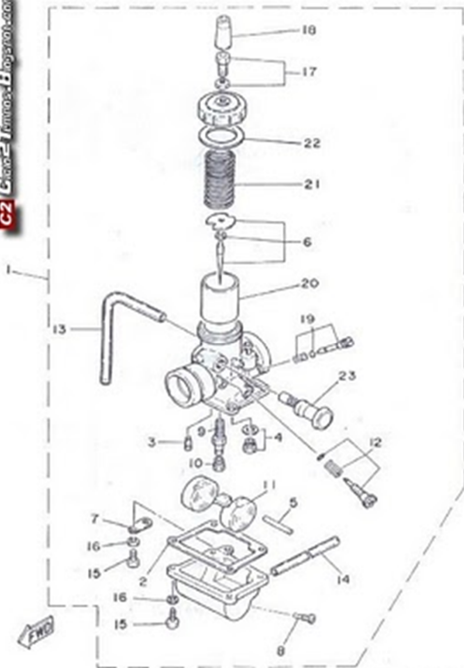
Carburador Rd135
