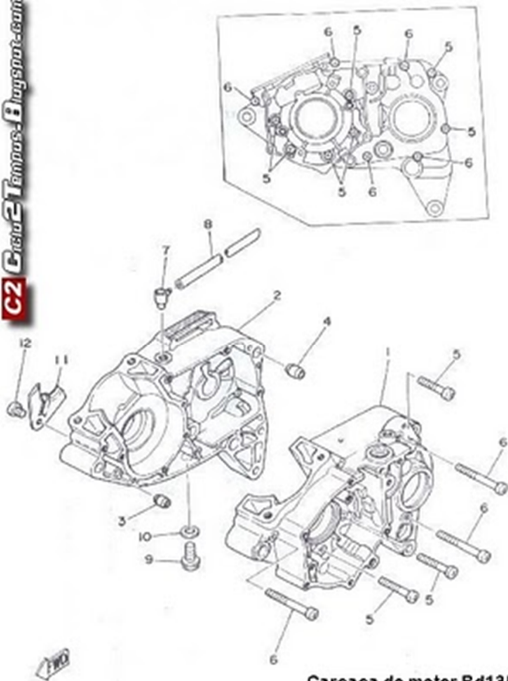
Carcaça do motor Rd135
